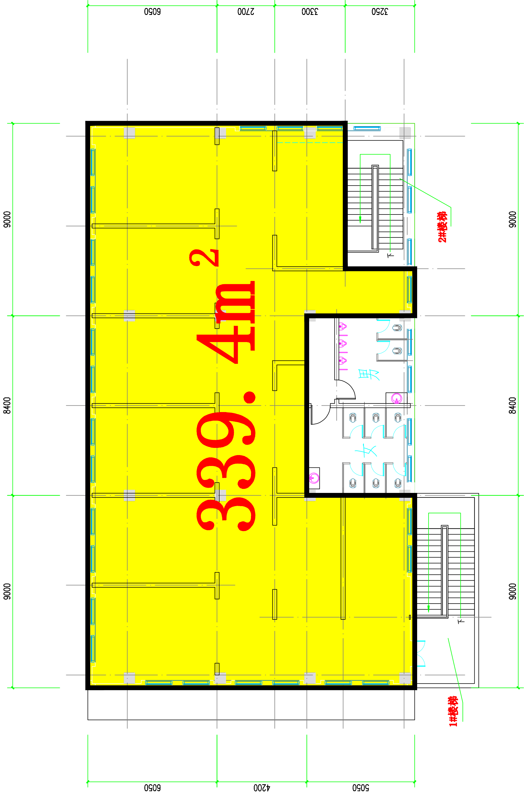
二层平面图
